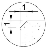
détail chanfrein
